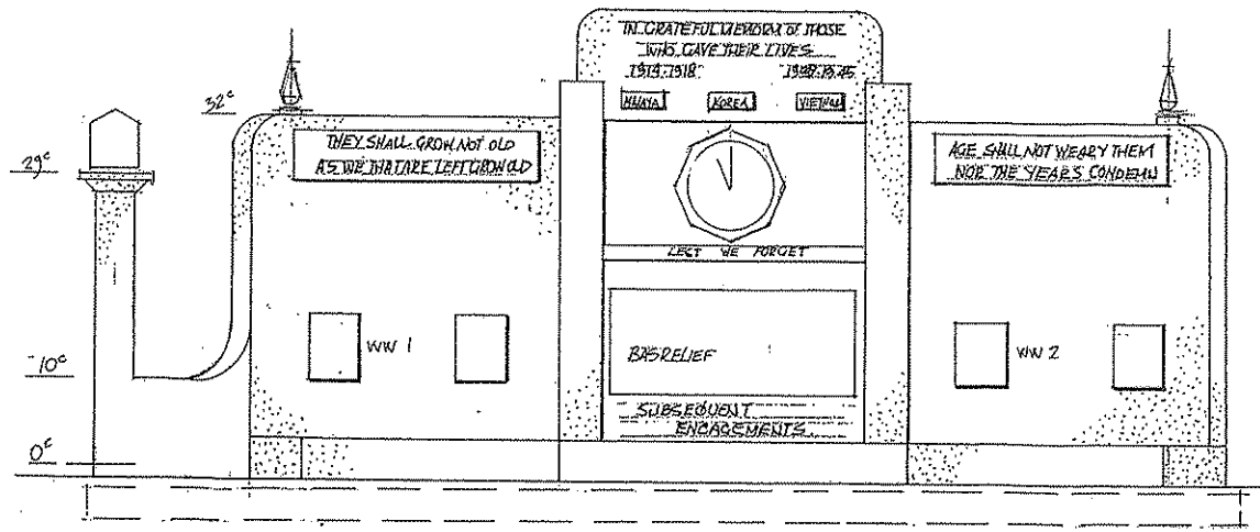
Elevation 1:50
